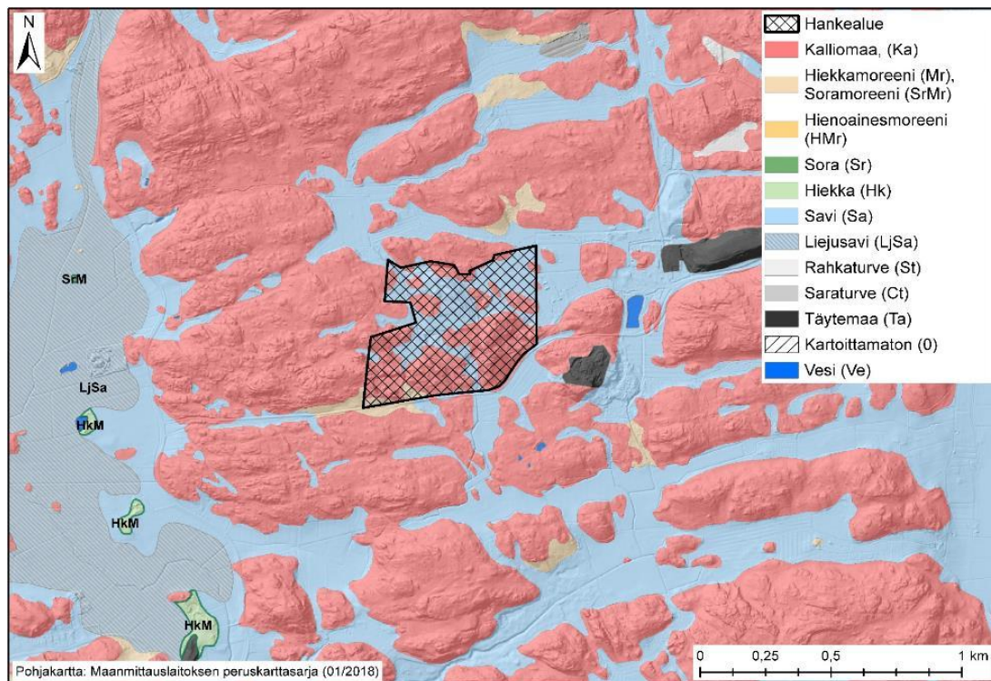
Kuva 5-5 Hankealueen maaperäolosuhteet.
