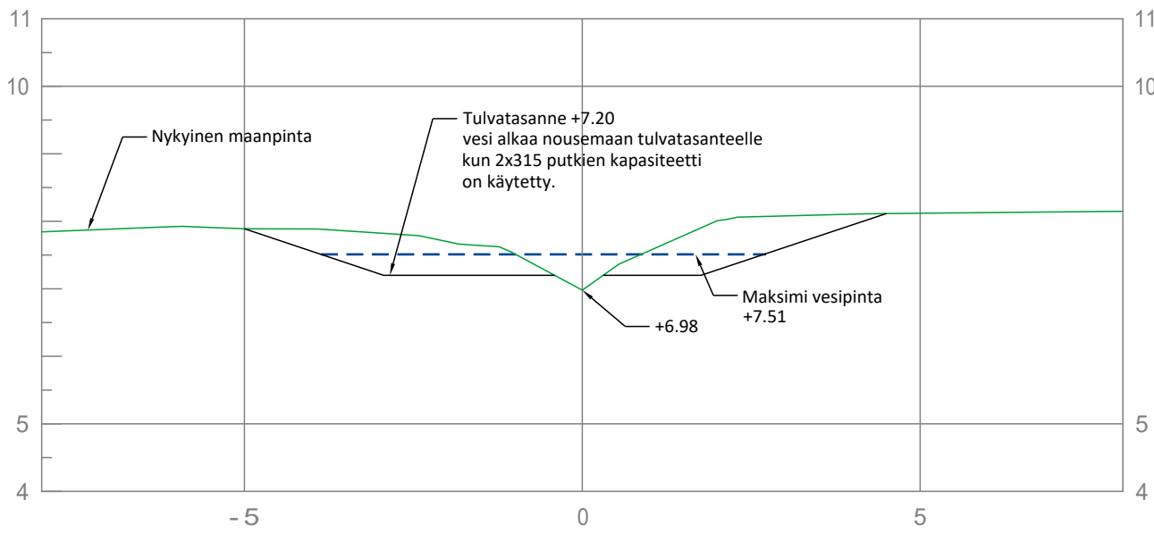
Leikkaus B-B Maapato ja alivirtausputket 1:100
