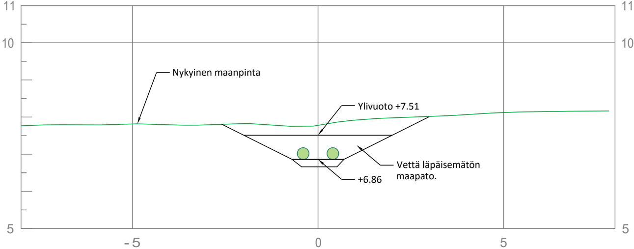
Leikkaus B-B Maapato ja alivirtausputket 1:100
