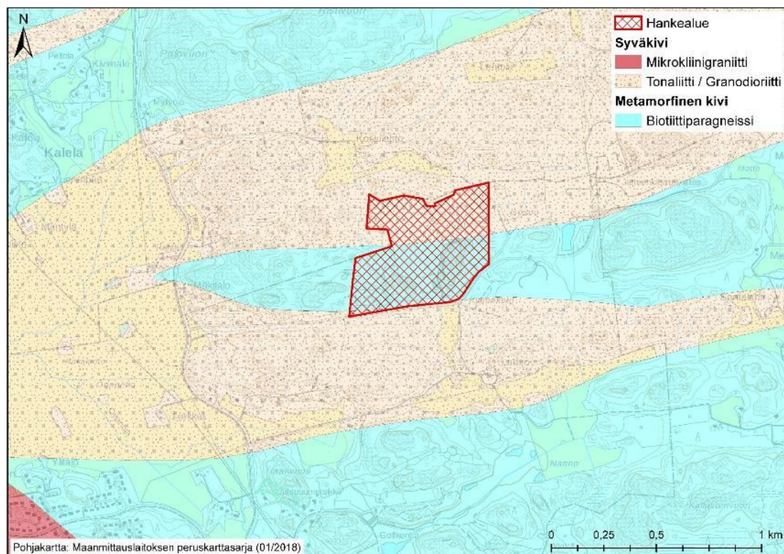
Kuva 5-6 Hankealueen kallioperäolosuhteet
